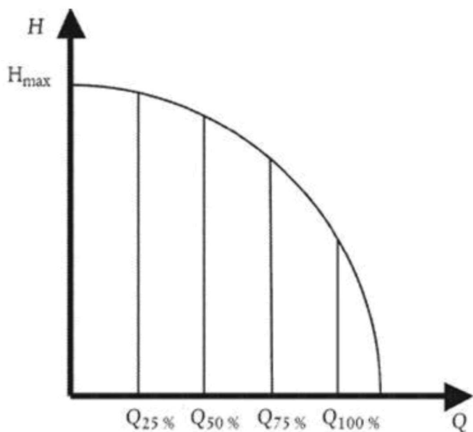
Рис. 3. Профиль нагрузки.
